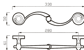
48 MN MANIGLIONE PULL HANDLE
