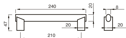
248 MN MANIGLIONE PULL HANDLE
