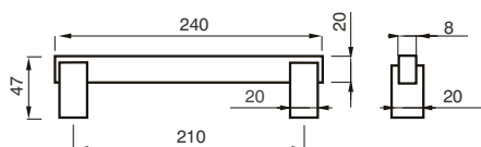
247 MN MANIGLIONE PULL HANDLE
