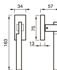
54 DK CREMONESE DK WINDOW HANDLE DK
