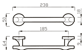
76 MN MANIGLIONE PULL HANDLE
