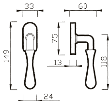
57 DK CREMONESE DK WINDOW HANDLE DK
