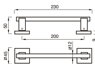
83 MNQ MANIGLIONE PULL HANDLE
