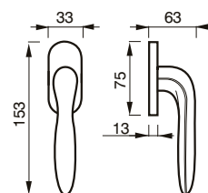
55 DK CREMONESE DK WINDOW HANDLE DK
