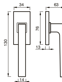
80 DK CREMONESE DK WINDOW HANDLE DK
