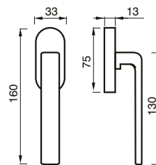
119 DKT CREMONESE DK WINDOW HANDLE DK
