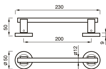
83 MN MANIGLIONE PULL HANDLE
