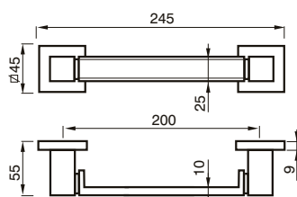
04 MN MANIGLIONE PULL HANDLE
