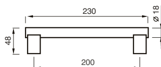
249 MN MANIGLIONE PULL HANDLE
