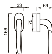
19 DK CREMONESE DK WINDOW HANDLE DK
