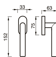
133 DK CREMONESE DK WINDOW HANDLE DK
