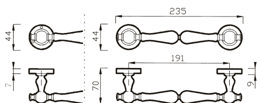
53 MNVV MANIGLIONE PULL HANDLE
