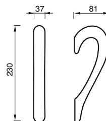
39 MN MANIGLIONE PULL HANDLE
