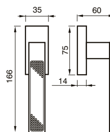
180 DK CREMONESE DK WINDOW HANDLE DK
