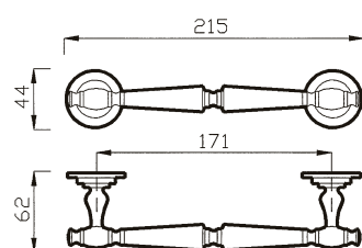
44 MNCV MANIGLIONE PULL HANDLE
