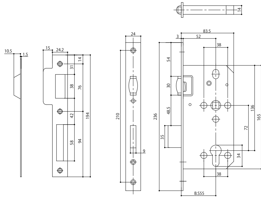
Cross Section Diagrams & Measurements for LLK Roller Latch Dead Lock LLKローラーラッチボルト 尺寸図/切欠図
