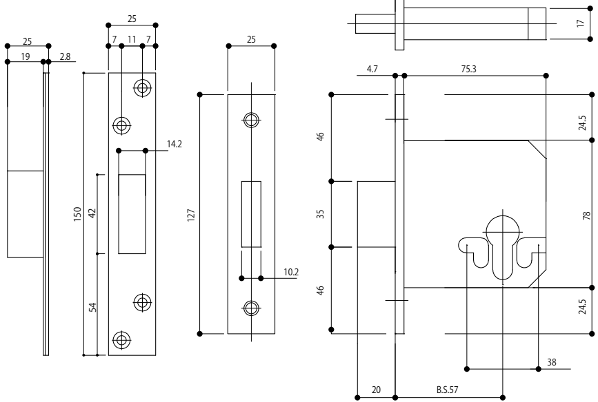
Fitting for Dead Bolt Lock デッドボルトのフィッティング
