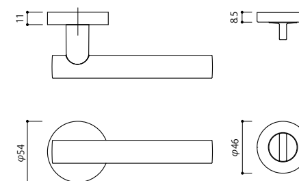
Measurements for Hotel Entrance Rose & Thumb Turn プレート・サムターンの寸法図
